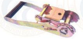
ITEM:EBRB053 A=52 B=52 C=230 BS: 2500KG/5500LBS
